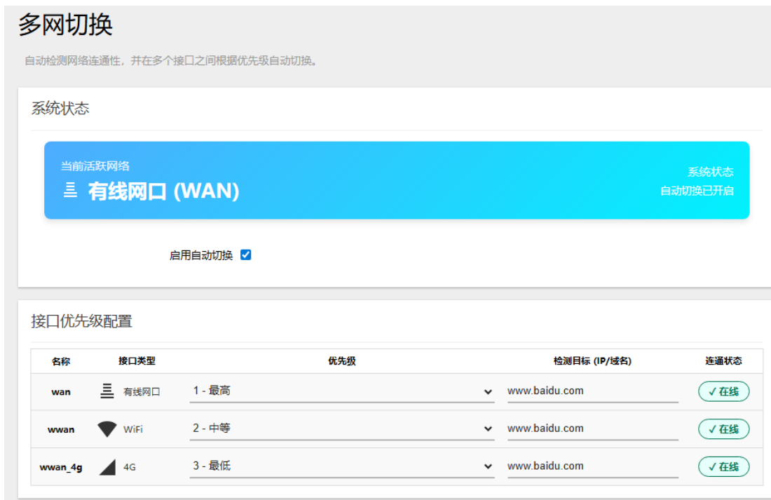
图 5.6 多网切换
