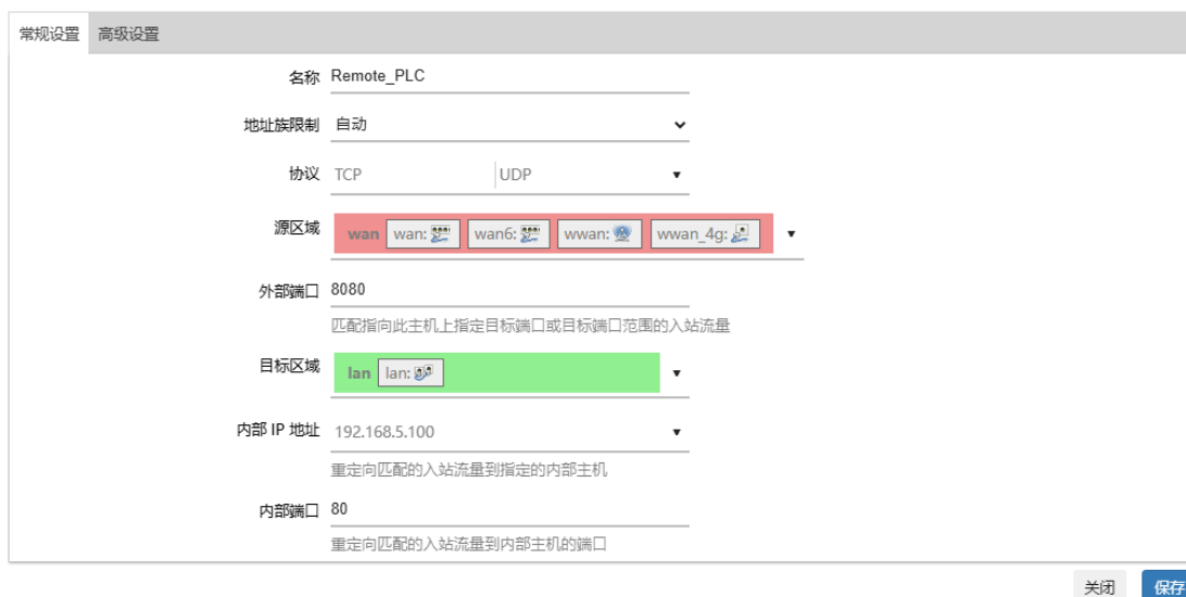
图 5.13 端口映射
