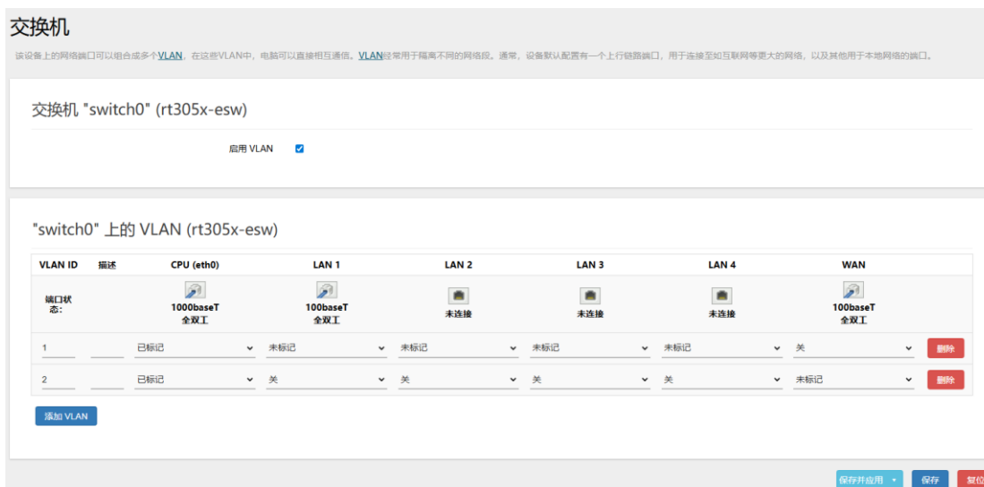
图 4.17 交换机
